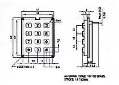
AK-304FM-diagram
