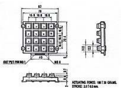
AK-1607-diagram
