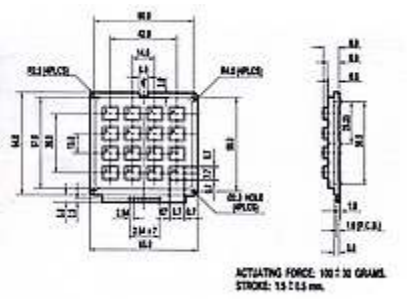
AK-1604-diagram
