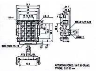
AK-507-diagram
